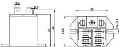
JQX-30F (PCB)外形尺寸
