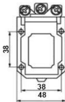
JQX-58F 1Z
